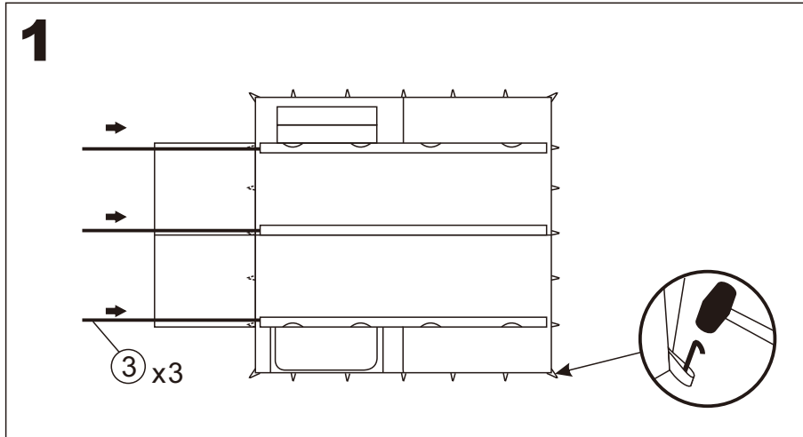
Flysheet
